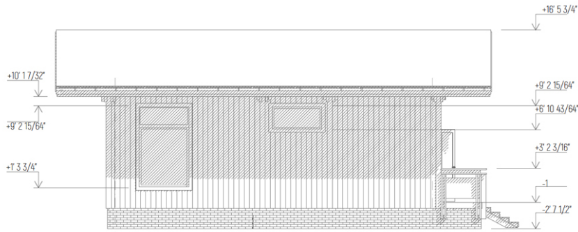
Elevation A-E
