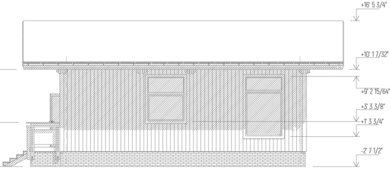
Elevation E-A
