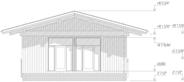
Elevation 1-5
