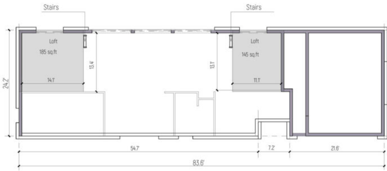
Loft plan
