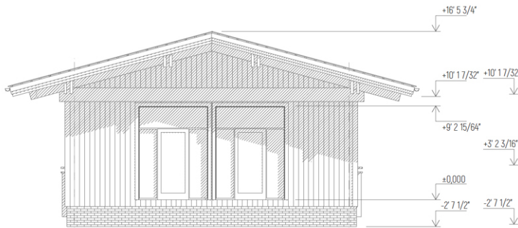
Elevation 1-5
