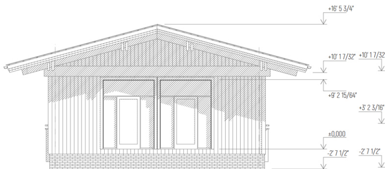
Elevation 1-5
