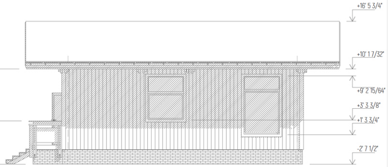
Elevation E-A
