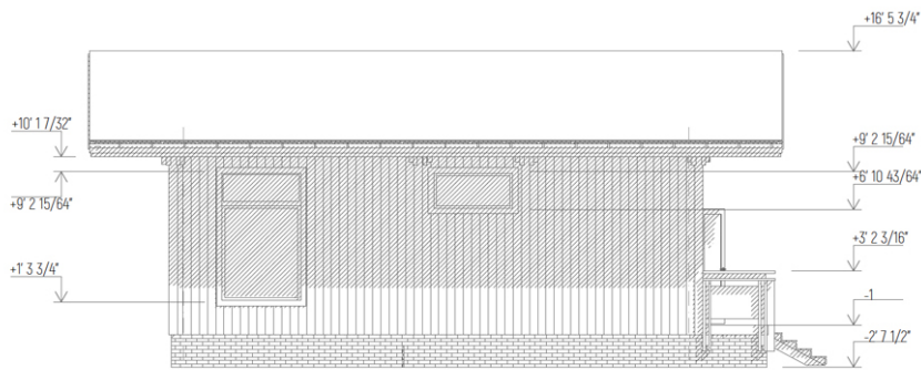
Elevation A-E
